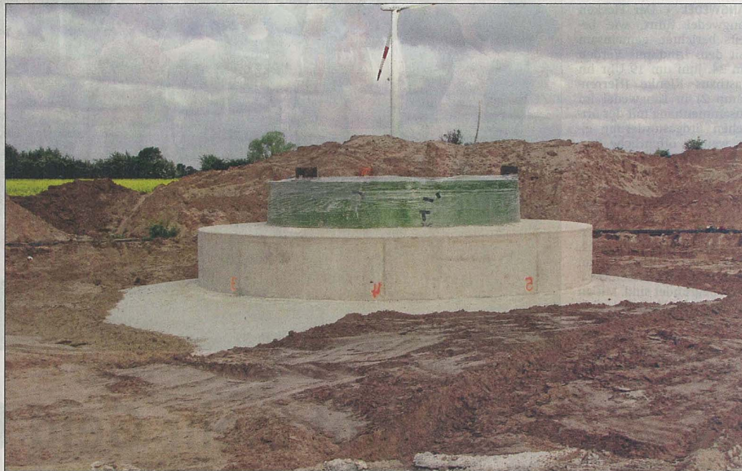
Das kreisrunde Fundament verrät: Hier (im Bereich Holtorf) wird in Kürze eine Windkraftanlage errichtet. • Foto: sp
